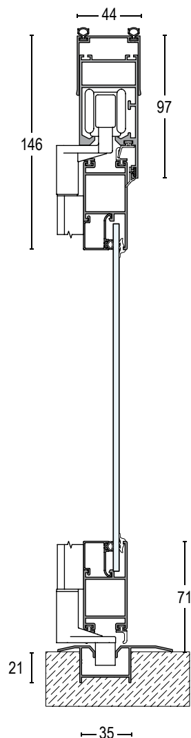
Guía empotrada
