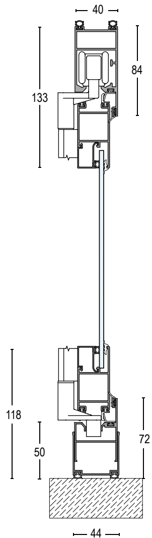
Guía superpuesta
